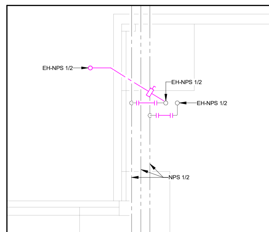
2 EXTRAIT M-250 1 : 50
