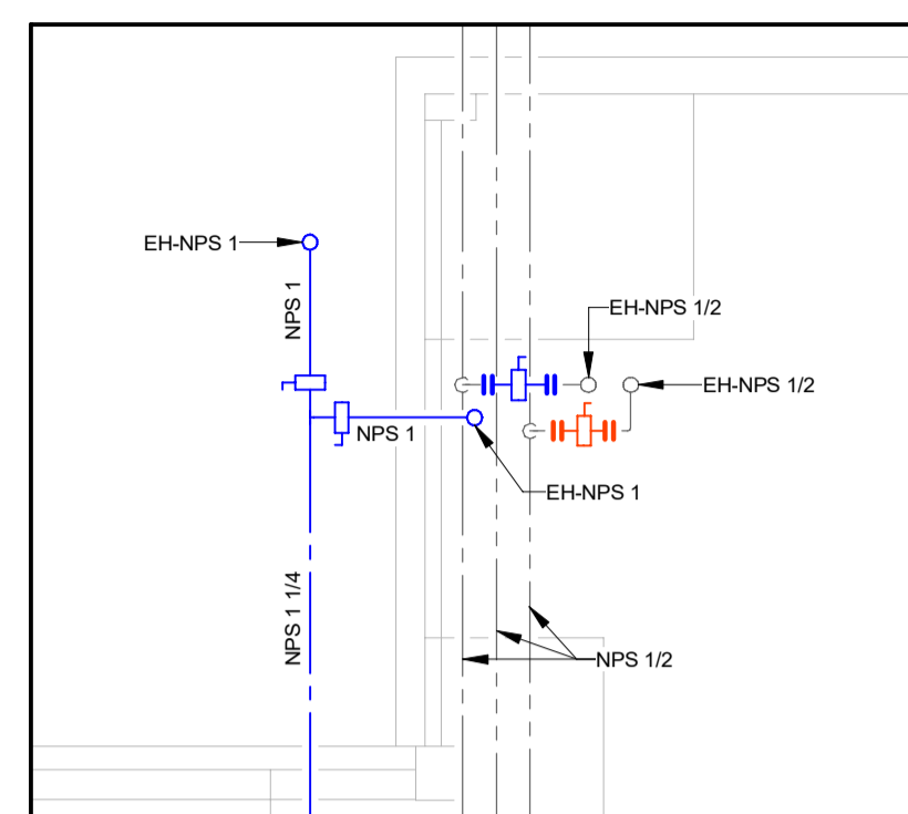
2 EXTRAIT M-251 1 : 50
